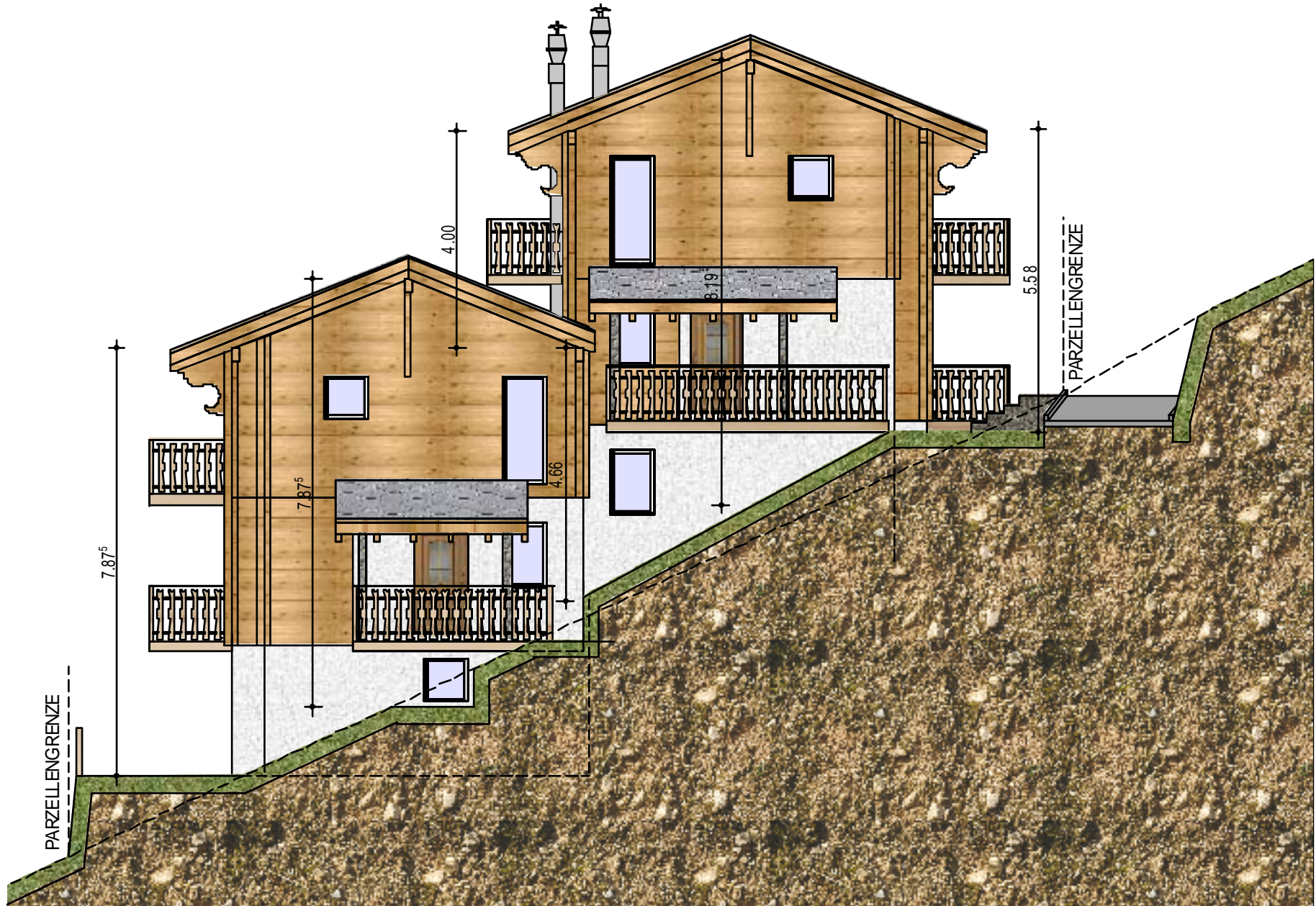
Nordfassade
