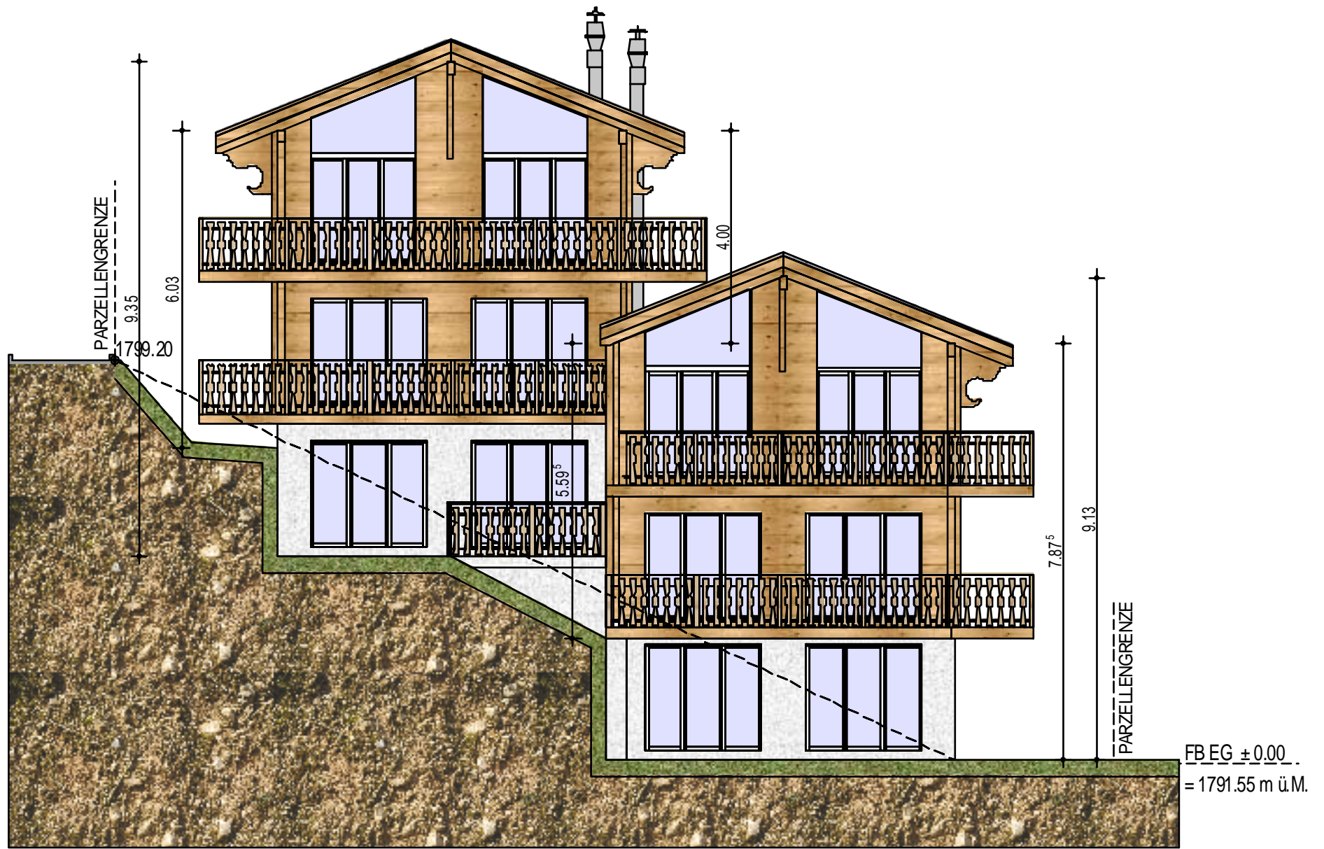
Südfassade
